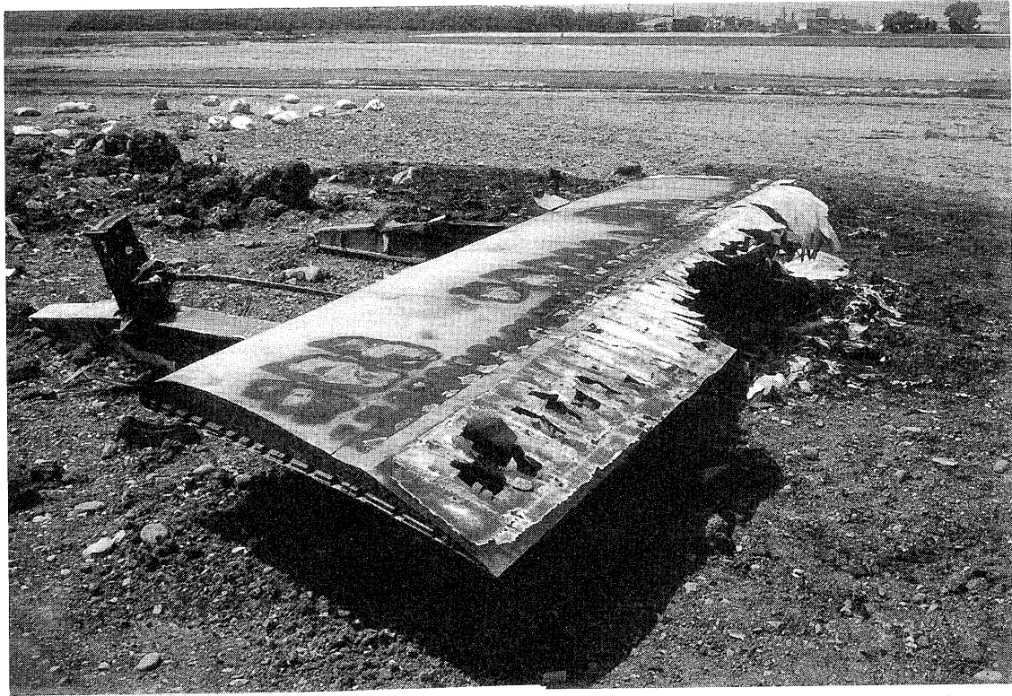
写真13 左センタ・フラップ
